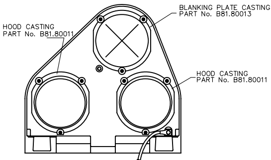
PL1R VERSION
